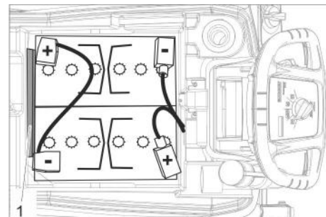
Акумуляторна батарея 6.654-290,0
