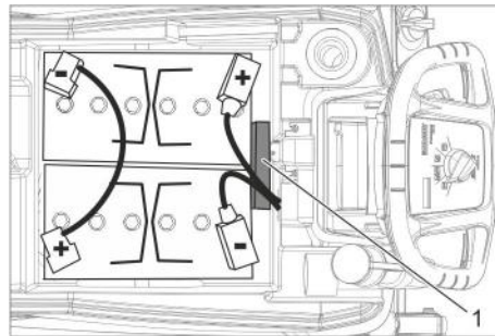
Batterie 6.654-141.0 1 Abstandshalter
