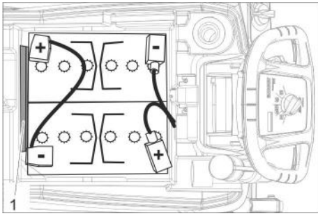
Аккумуляторная батарея 6.654-290,0
